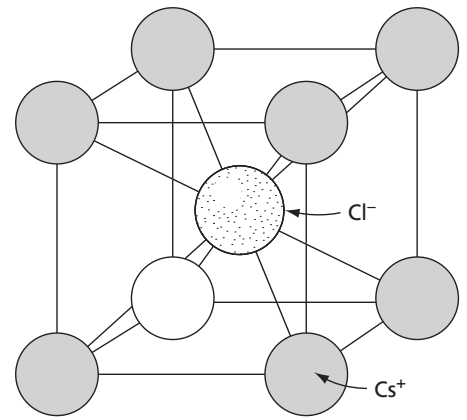
FIG. 3.2 The cesium chloride lattice
